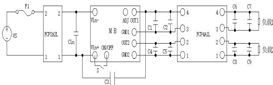
F1:4A保险丝（快熔）
