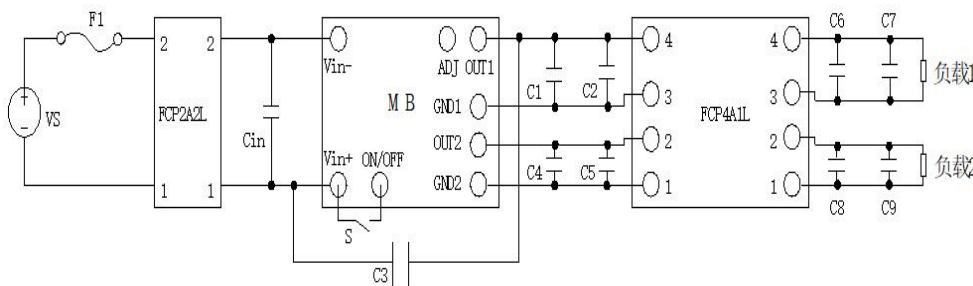
F1: 4A保险丝（快熔）
